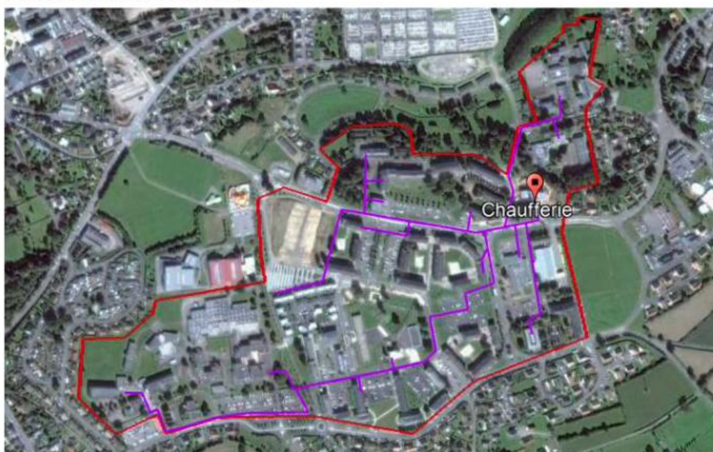
Figure 1 : périmètre et tracé du réseau de chaleur
