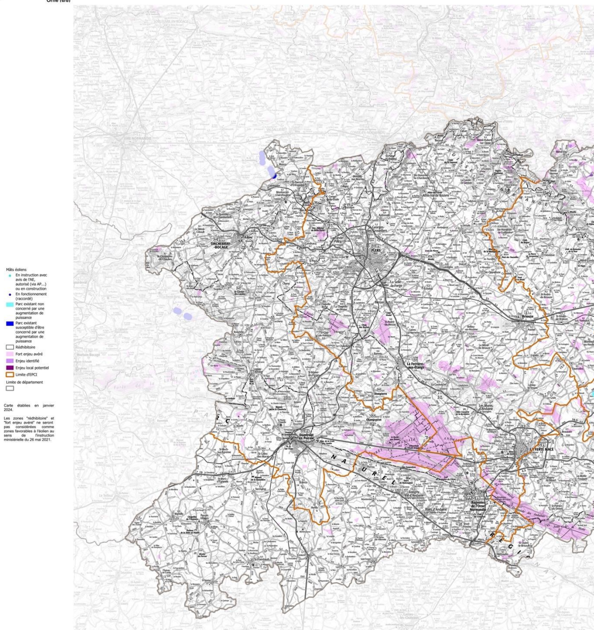
Identification des zones potentiellement favorables à l'éolien en Normandie : niveaux d'enjeux des différentes thématiques (biodiversité, paysage, contraintes techniques) du département. Orne (6/8)
