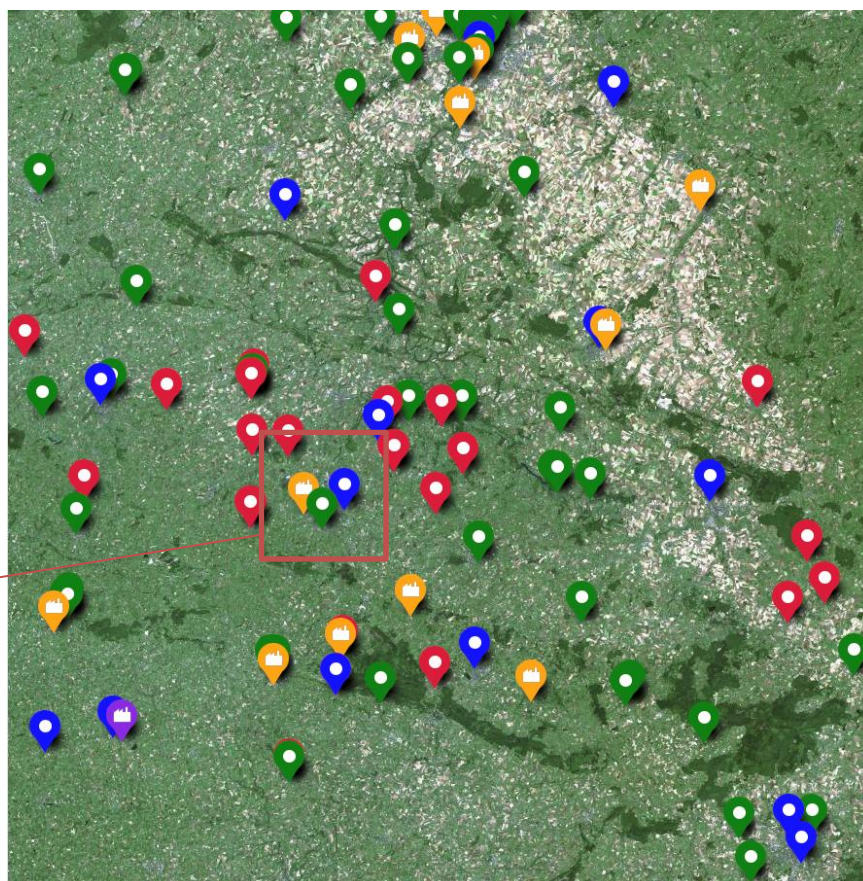
Cartographie des chaufferies bois collectives et industrielles normandes fin 2022 par Biomasse_Normandie
